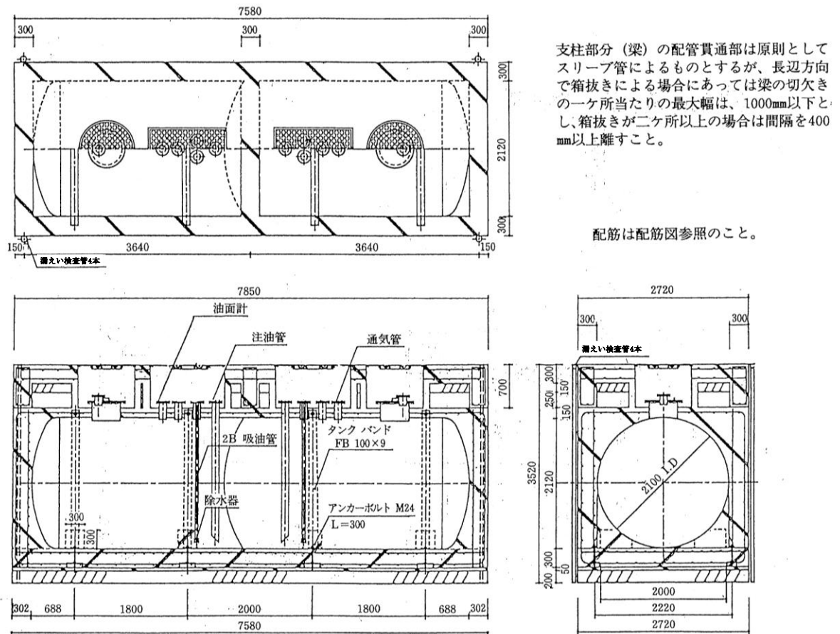
第4-3-7図 コンクリート被覆タンク埋設図 (20kl 中仕切 10:10 直径2.1m)
