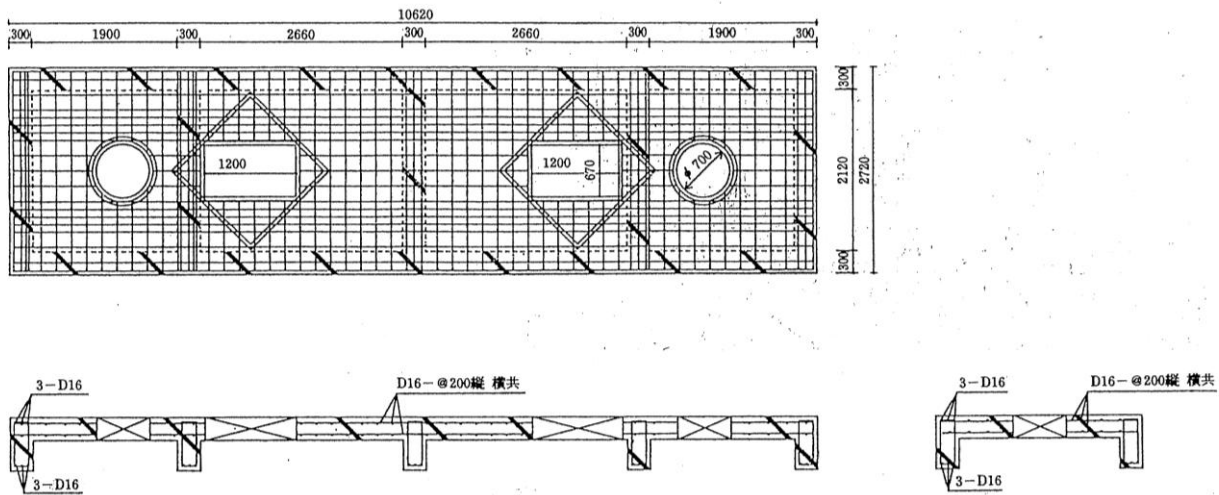
第4-3-4図 コンクリート被覆タンク配筋図 (30k1 中仕切 15:15 直径2.1m)
