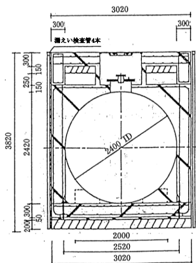
第4-3-5図 コンクリート被覆タンク埋設図 (20k1 中仕切 10:10 直径2.4m)
