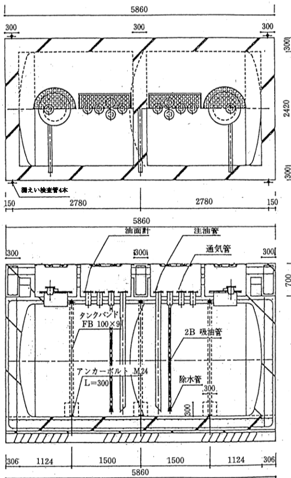
第4-3-4図 コンクリート被覆タンク配筋図 (30k1 中仕切 15:15 直径2.1m)
