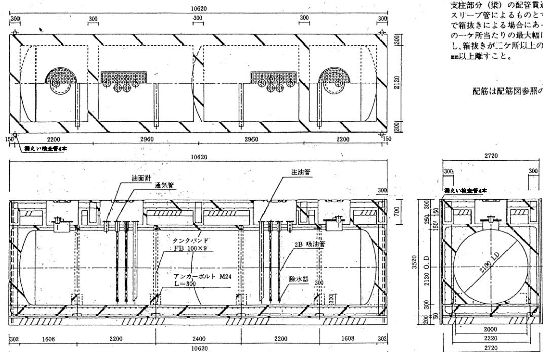
第4-3-3図 コンクリート被覆タンク埋設図 (30kl 中仕切 15:15 直径2.1m)
