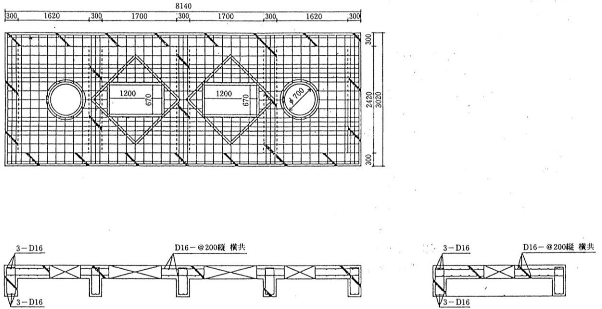
第4-3-2図 コンクリート被覆タンク配筋図 (30kl 中仕切 15:15 直径2.4m)
